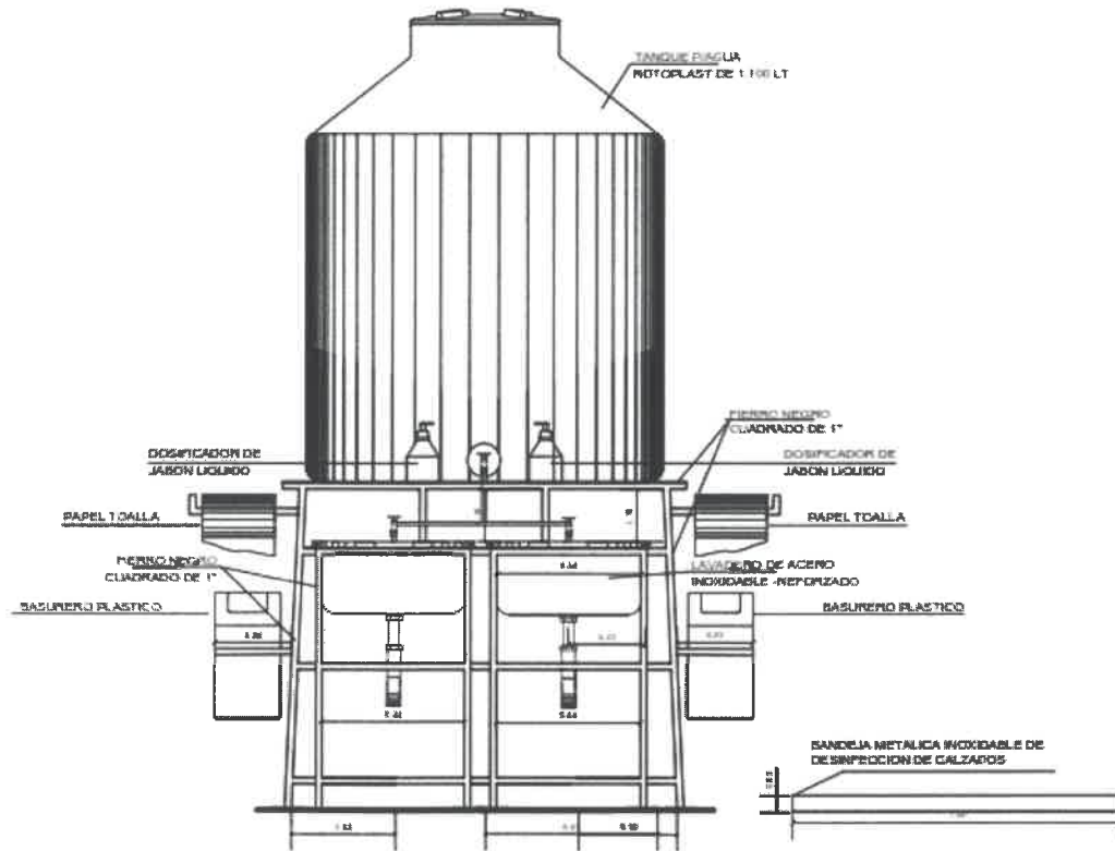
ELEVACION FRONTAL
